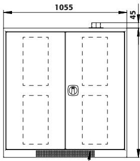
Ventilation naturelle
