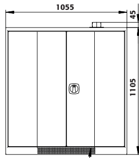
Ventilation naturelle
